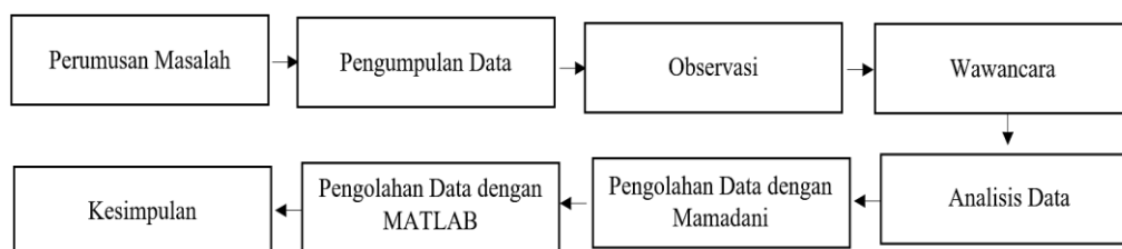
Gambar 1. Kerangka Penelitian
