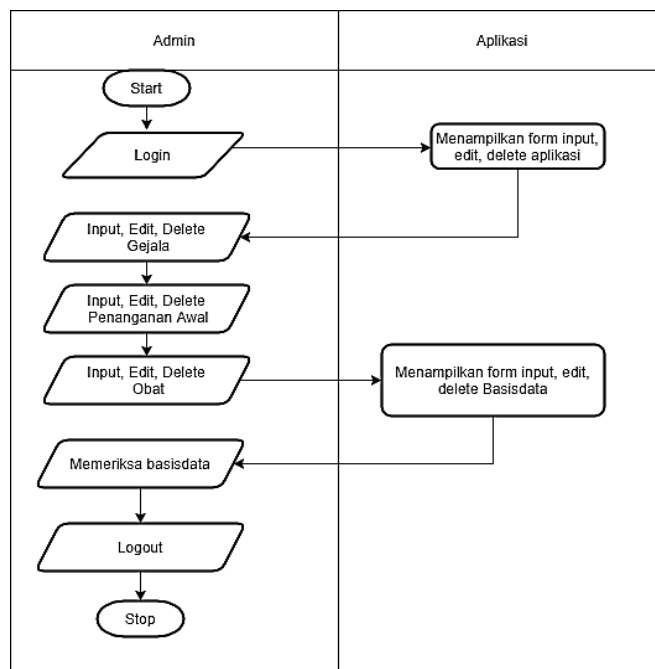
Gambar 5. Diagram aktivitas admin
