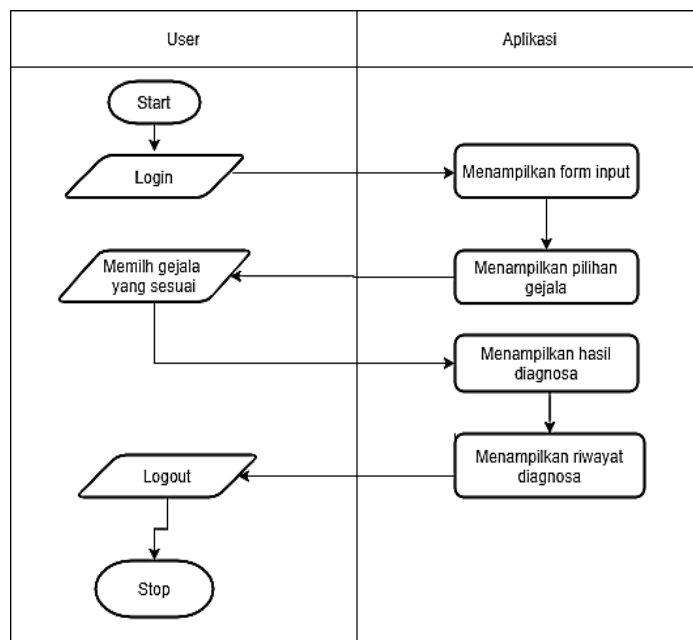
Gambar 4. Diagram aktivitas user
