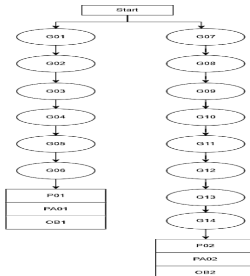
Gambar 7. Pohon keputusan
