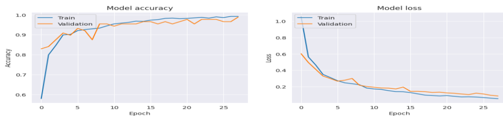
Gambar 5. Grafik Rasio 90/10
