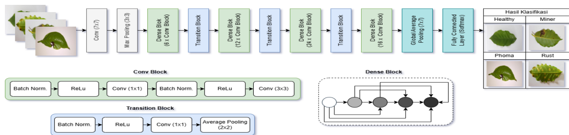
Gambar 4. Alur Arsitektur DenseNet121
