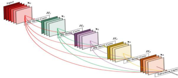
Gambar 3. Arsitektur DenseNet121
