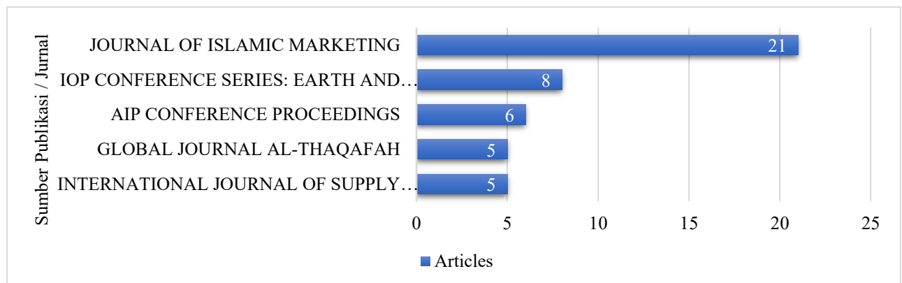
Gambar 3. Lima Jurnal Paling Produktif
