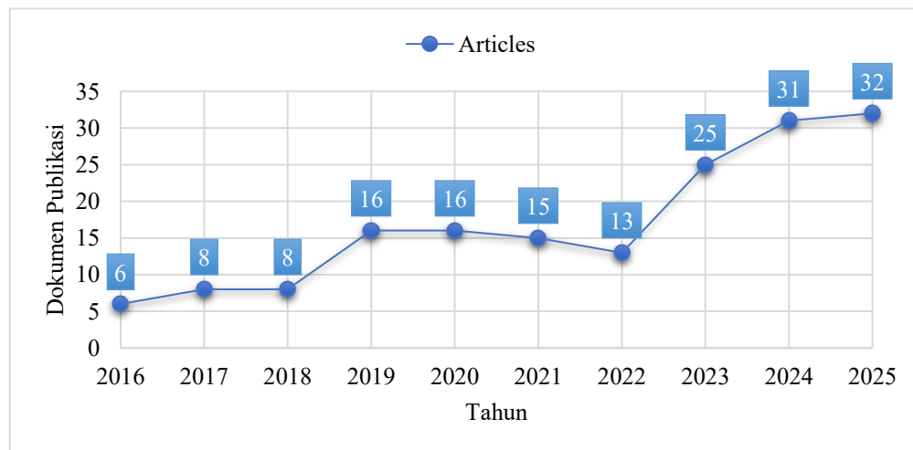
Gambar 2. Tren Publikasi Tahunan Penelitian Sertifikasi Halal Periode 2016–2025
