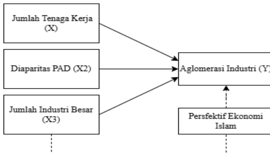
Gambar 2. Kerangka berpikir
