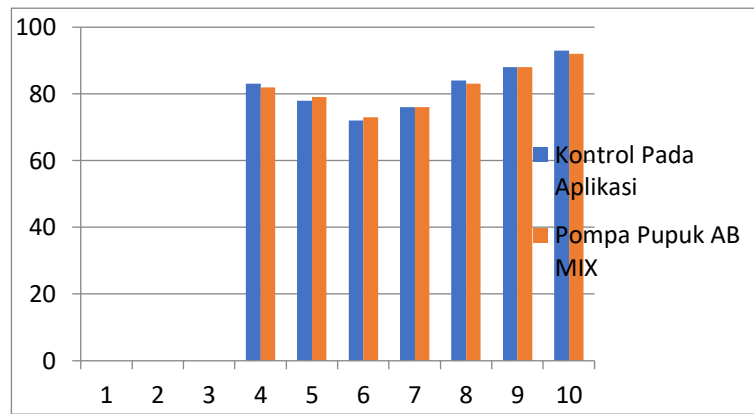
Gambar 3. Grafik pembacaan Suhu Sensor DHT22
