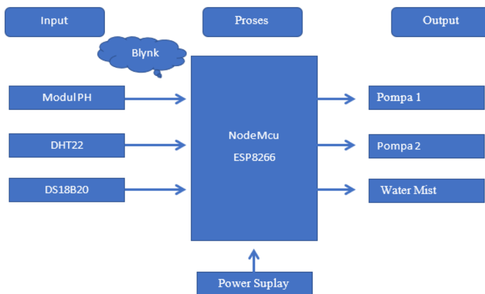
Gambar 1. Blok Perancangan Sistem
