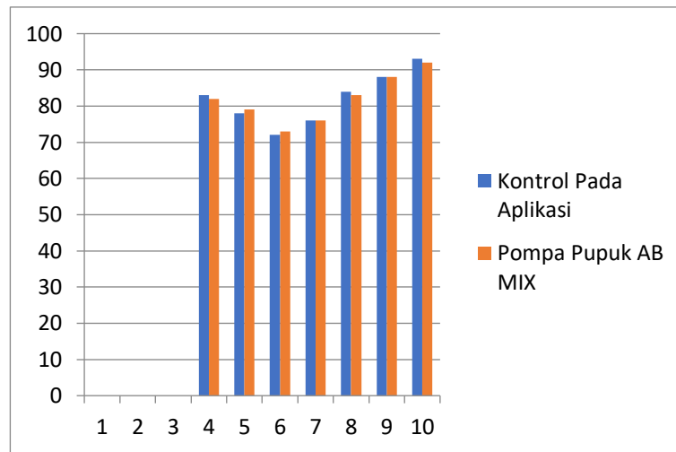
Gambar 4. Grafik pembacaan Kelembaban Sensor DHT22
