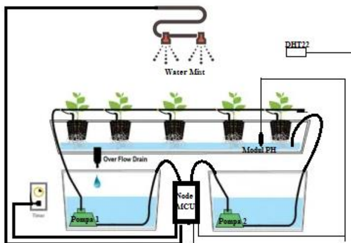
Gambar 2. Blok Perancangan Sistem
